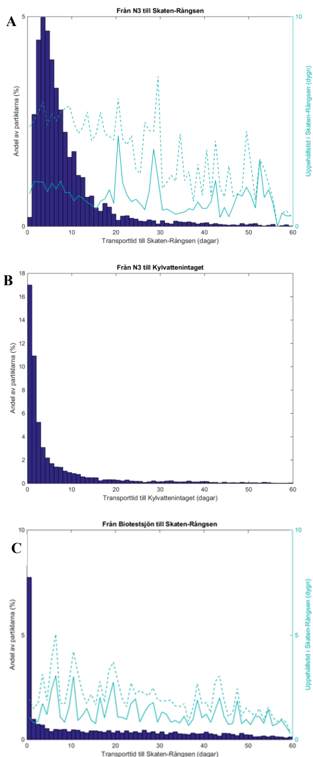
Figur 4-5. Histogrammen beskriver ett exempel på fördelningen av transporttiden för partiklarna från en av utsläppskällorna (N3) direkt till Natura 2000-området Skaten-Rångsen via Dyviksfjärden (A), eller genom att partiklarna sugas in i kylvattenkanalen (B) och släpps ut via Biotestsjön och vidare mot Natura 2000-området Skaten-Rångsen (C). Linjerna visar den genomsnittliga uppehållstiden i området för partiklar med en viss transporttid. Den heldragna linjen visar den genomsnittliga uppehållstiden vid första besöket för partiklar med en viss transporttid, medan den streckade linjen även inkluderar uppehållstiden om partikeln transporteras tillbaka in i området vid ett eller flera senare tillfällen (inom 60 dagar från utsläppstiden).
