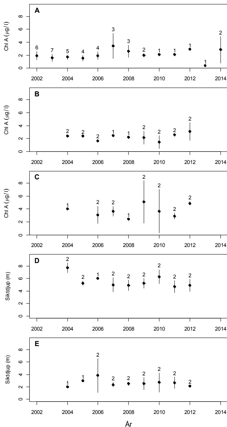
Figur 3-9. Överst, sommarmedelvärden (juni–september) för koncentrationen av olika kväveformer i Asphällsfjärden, samt N/P-kvoter för löst oorganiskt och totalhalter. Nederst, sommarmedelvärden för klorofyll A och siktdjup i Asphällsfjärden (A), Öregrundsgrepen (B, D) och Kallrigaffjärden (C, E). De lodräta staplarna visar standardavvikelsen för observationerna och siffran ovanför är antalet observationer. Data från Asphällsfjärden är från SKB:s mätningar och data från Öregrundsgrepen och Kallrigaffjärden kommer från Svealands Kustvattenförbunds mätningar.
