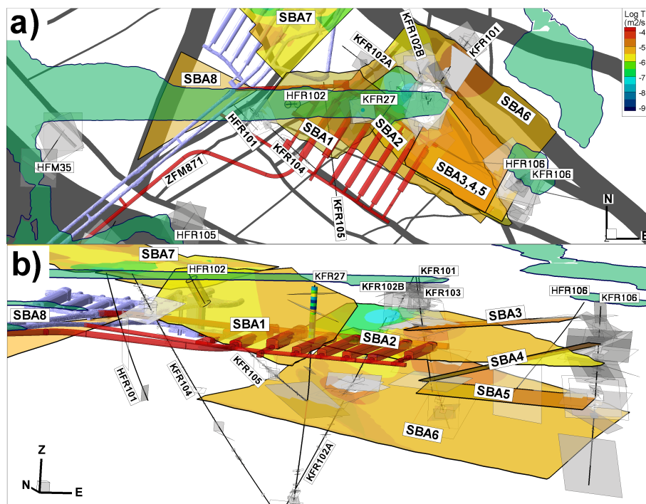
Figur 3-1. De åtta SBA strukturerna som de presenteras i den hydrogeologiska modellen tillsammans med försvarslayout L0. Figur a) uppfifrån, b) från sidan mot nordost. Färgen på SBA strukturerna återspeglar deras antagna transmissivitet utifrån borrhålstransmissivitet.
