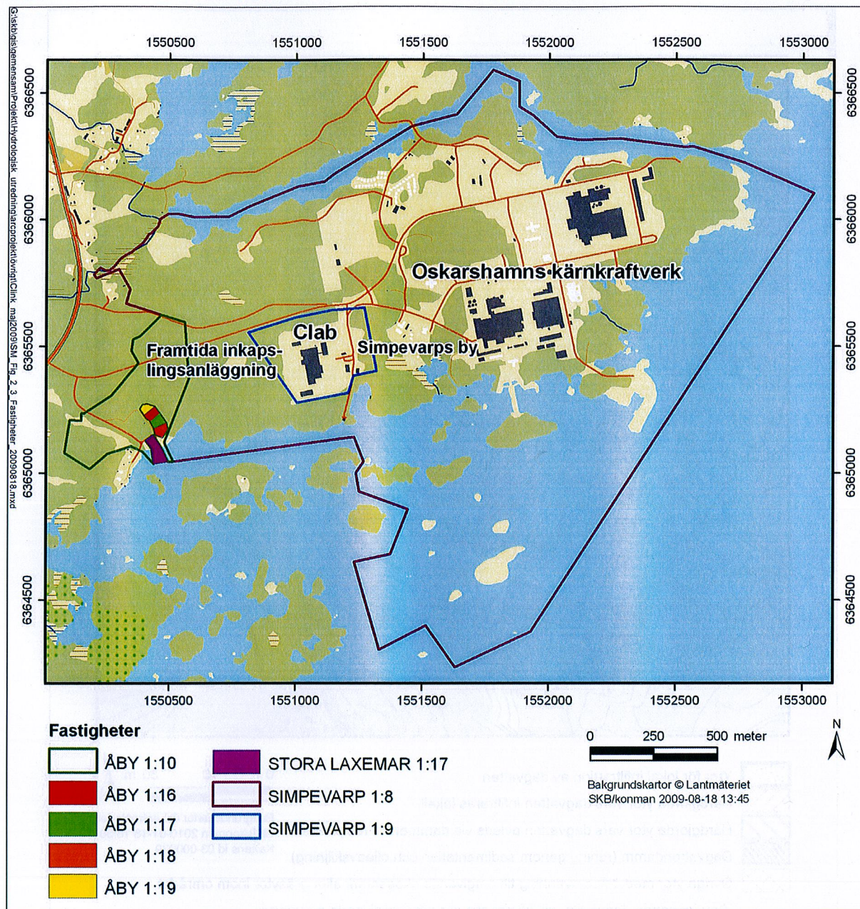
Figur 1. Fastigheter och byggnader i Clabs omgivning. Kartan visar även läget för inkapslingsanläggningen, som kommer att uppföras i direkt anslutning till Clab.
